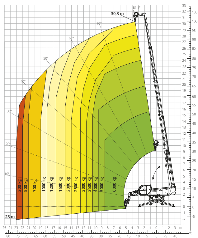
Abaque de charge avec TREUIL 6 000 kg ATT - 02 - 004
