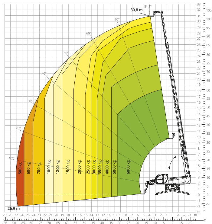
Abaque de charge avec STABILISATEURS DÉPLOYÉS 360° ATT-03-004
