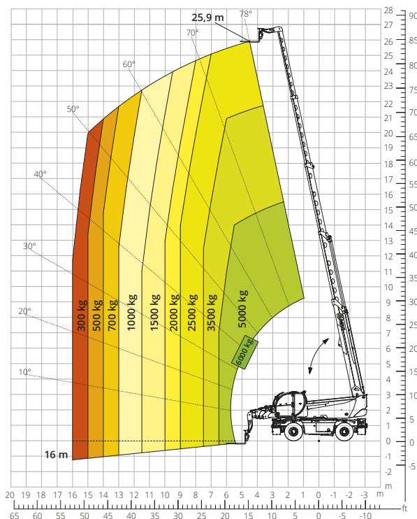
Abaque de charge FRONTAL SUR PNEUS ATT-03-004
