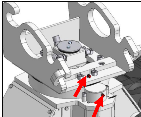
Fig. 10: Smeerpunten op draaikrans
