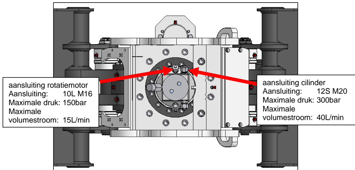
Fig. 8: Hydrauliek-aansluitingen
