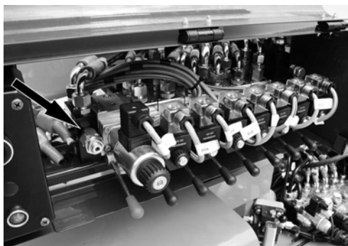
Fig. 8 Overdrukklep hoogwerkerdeel
